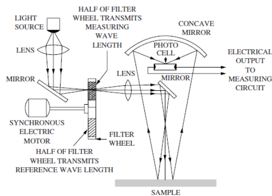
Figura 5 - Esquemático funcional de um medidor de umidade por infravermelho (LIPTÁK & BRODGESELL, 2003).
