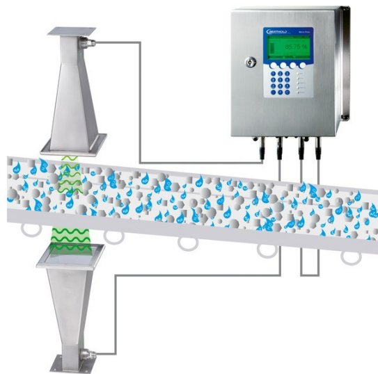
Figura 4 - Sistema de medição de umidade por micro-onda (Contactless Measurement of Water Content and Moisture, 2004).
