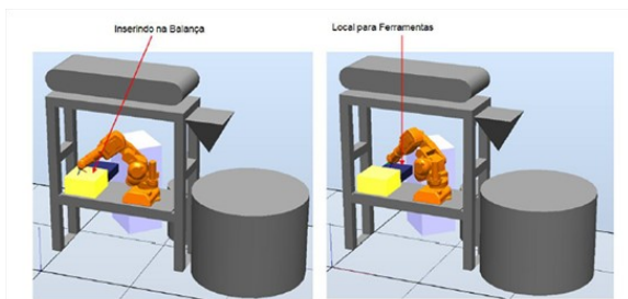
Figura 10 - Estudo de leiaute com maquete 3D.
